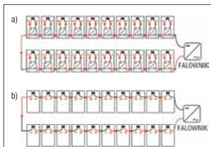
Rys. 4. Porównanie systemu fotowoltaicznego o mocy 6 kWp z 20 modułami pod względem połączeń wtykowych DC: a) system z optymalizatorami; 61 połączeń, b) system z tradycyjnym falownikiem łańcuchowym; 21 połączeń
